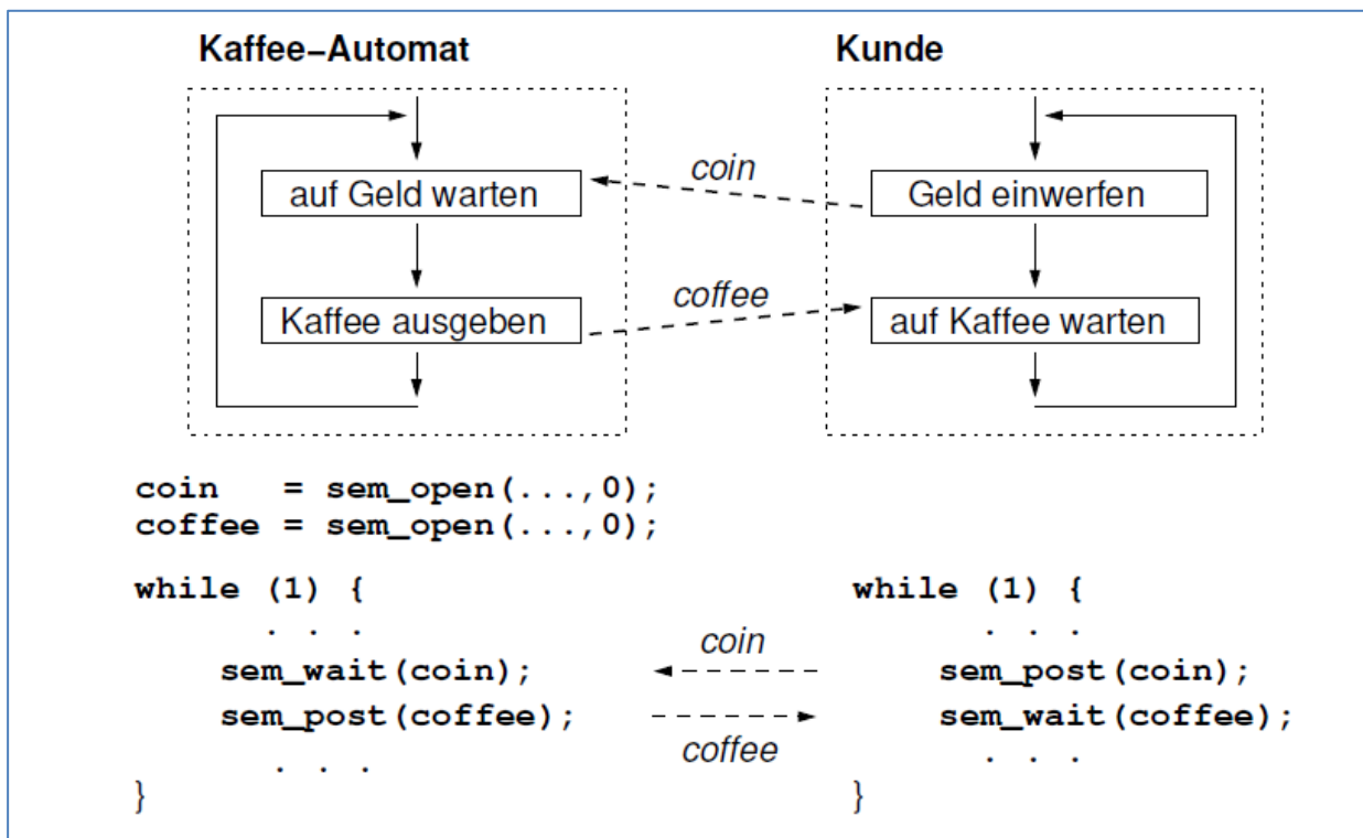
Abbildung 1: Ablaufgraph und Pseudocode für 2 Prozesse und zwei Semaphore
